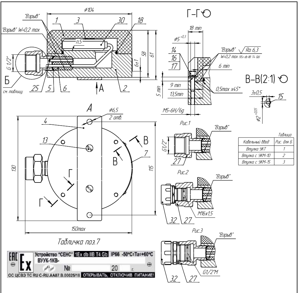
Рисунок В.1 – Чертеж средств взрывозащиты
